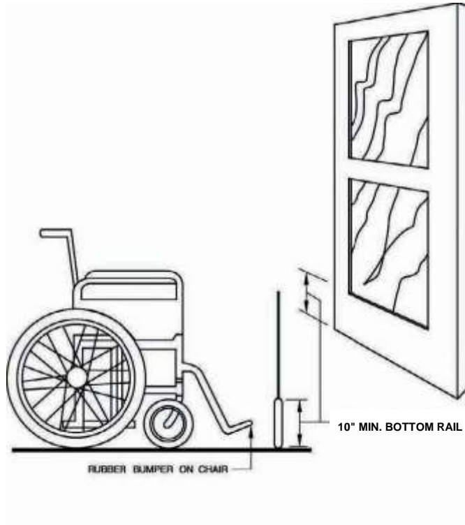
DOOR CONSTRUCTION
